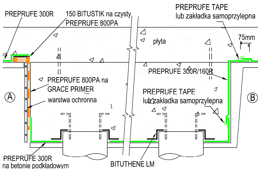
DETAL OCZEPU - PEŁNE ZABEZPIECZENIE
