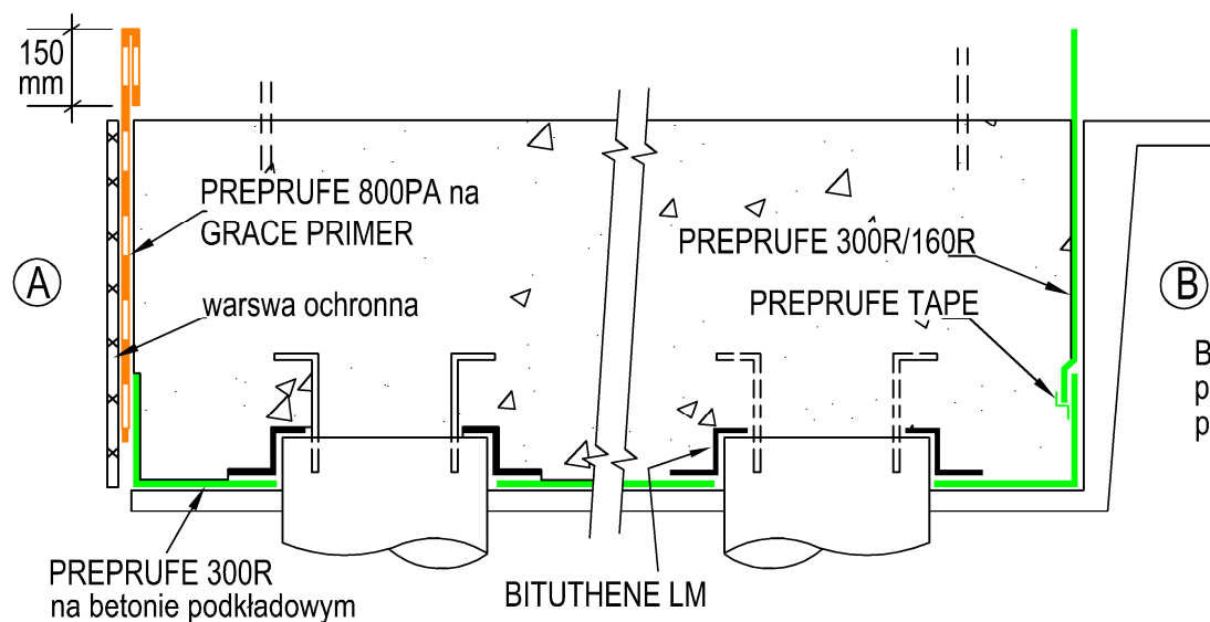
DETAL OCZEPU - PEŁNE ZABEZPIECZENIE
