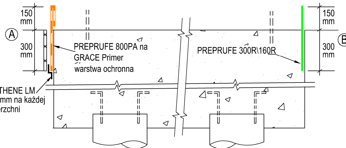
OCZEP MONOLITYCZNY - NIECIĄGŁOŚĆ HYDROIZOLACJI ① DOTYCZY TYLKO OCZEPÓW PALI POWYŻEJ 600mm GŁĘBOKOŚCI
