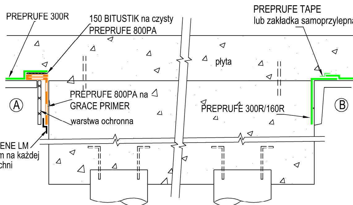
OCZEP MONOLITYCZNY - NIECIĄGŁOŚĆ HYDROIZOLACJI ② DOTYCZY TYLKO OCZEPÓW PALI POWYŻEJ 600mm GŁĘBOKOŚCI
